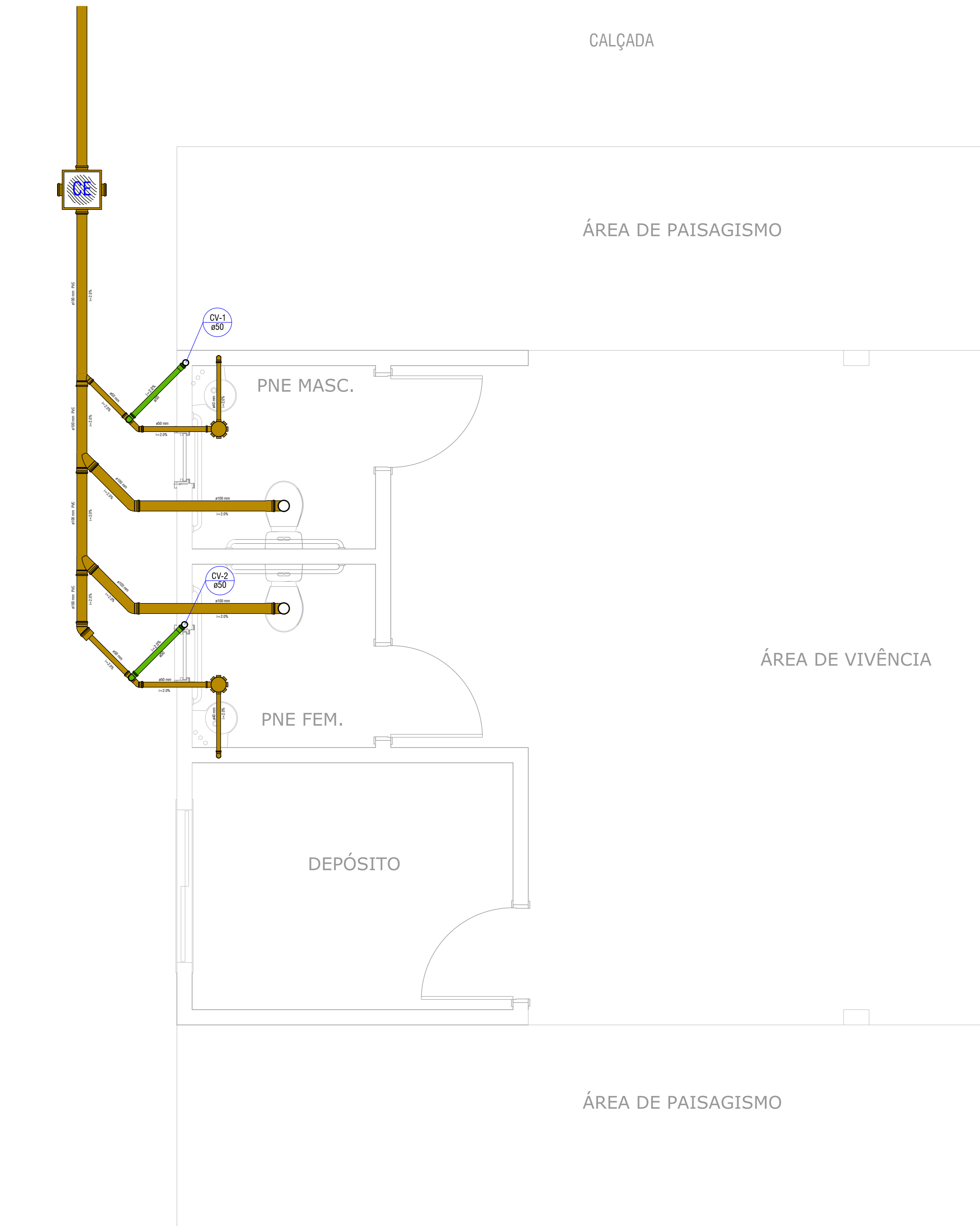
Detalhe ESGOTO - GERAL escala 1:25
