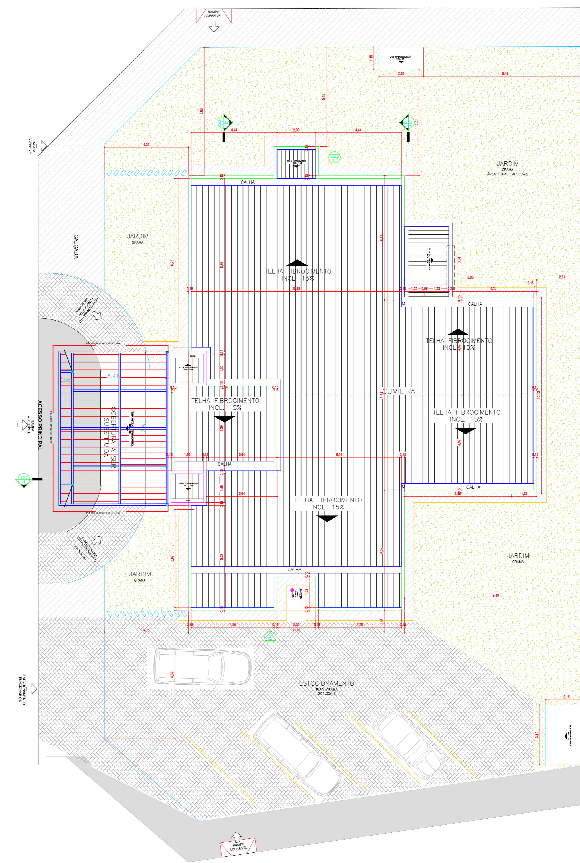
PLANTA DE COBERTURA / IMPLANTAÇÃO ESC. 1:100
