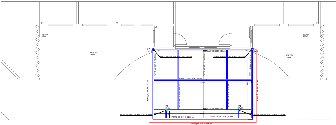
Planta Baixa Estrutura Metálica da Cobertura escala 1:50
