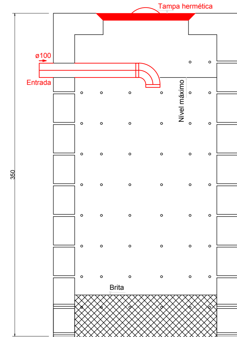
SUMIDOURO - CORTE S/ ESC.
