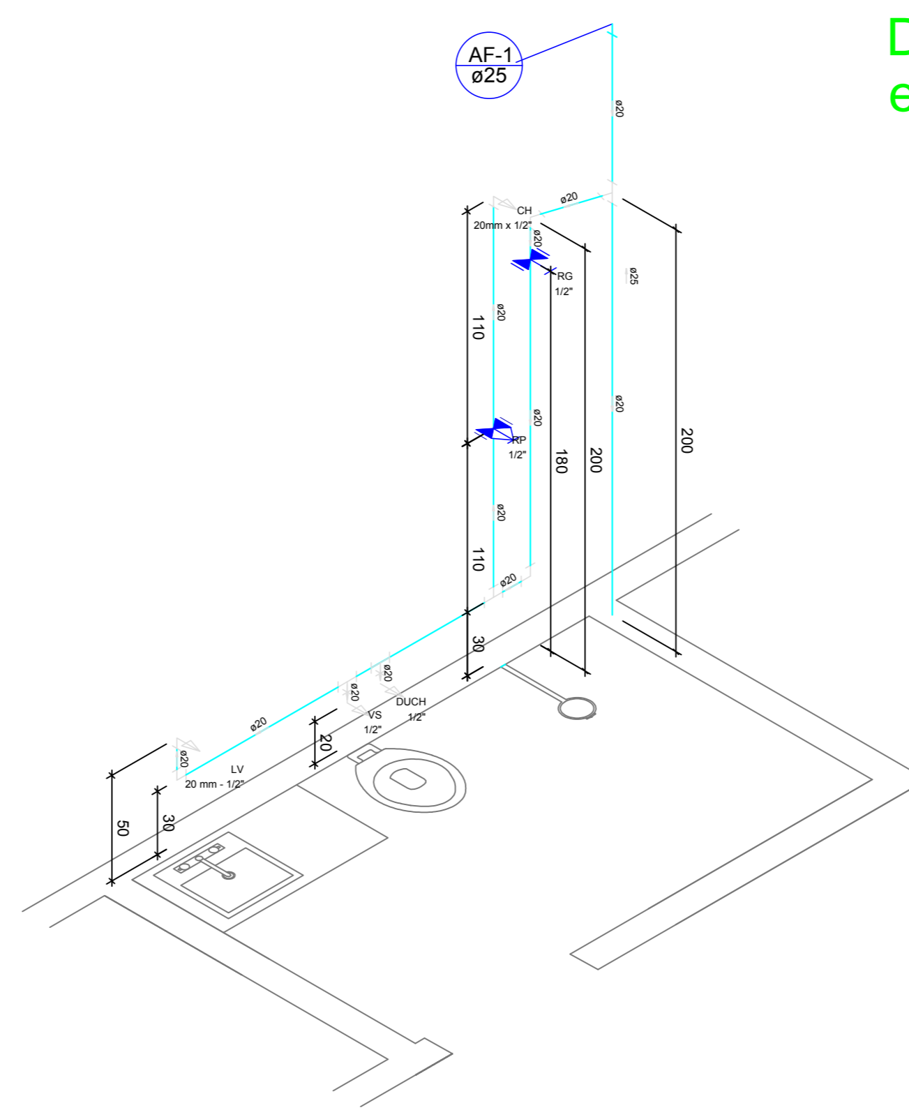
Detalhe ISOMÉTRICO BANHEIROS MASCULINOS E FEMININOS escala 1:25
