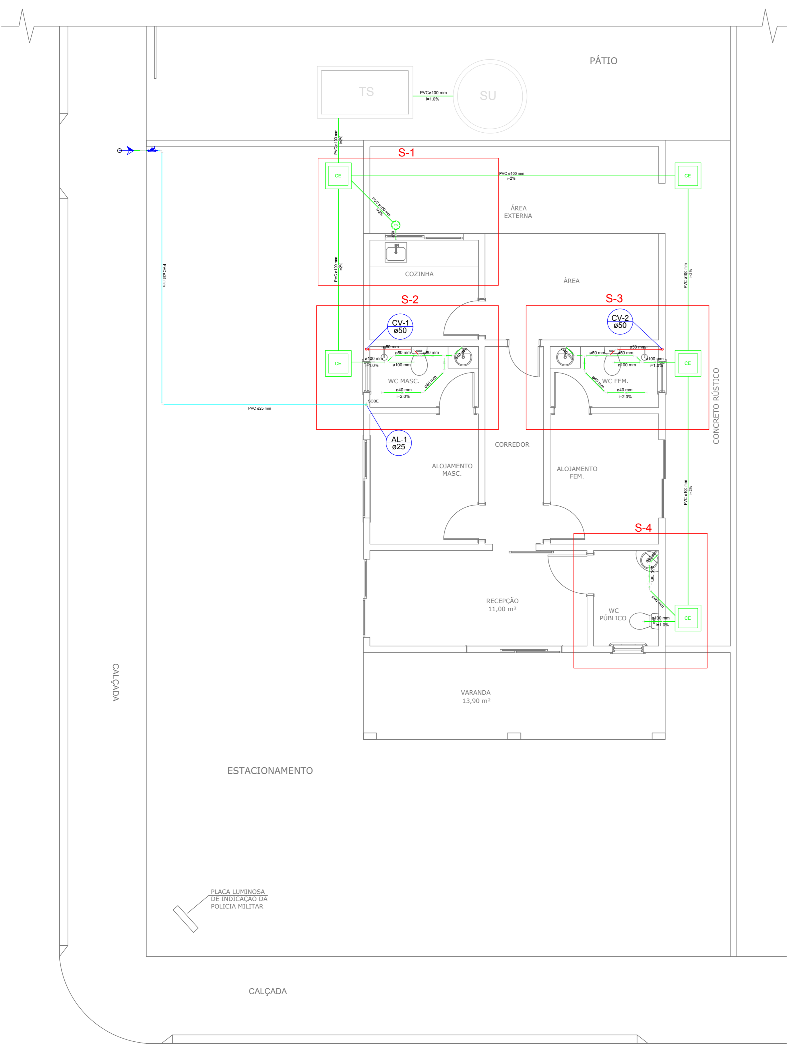
PLANTA BAIXA - IMPLANTAÇÃO GERAL REDE DE ESGOTO escala 1:50
