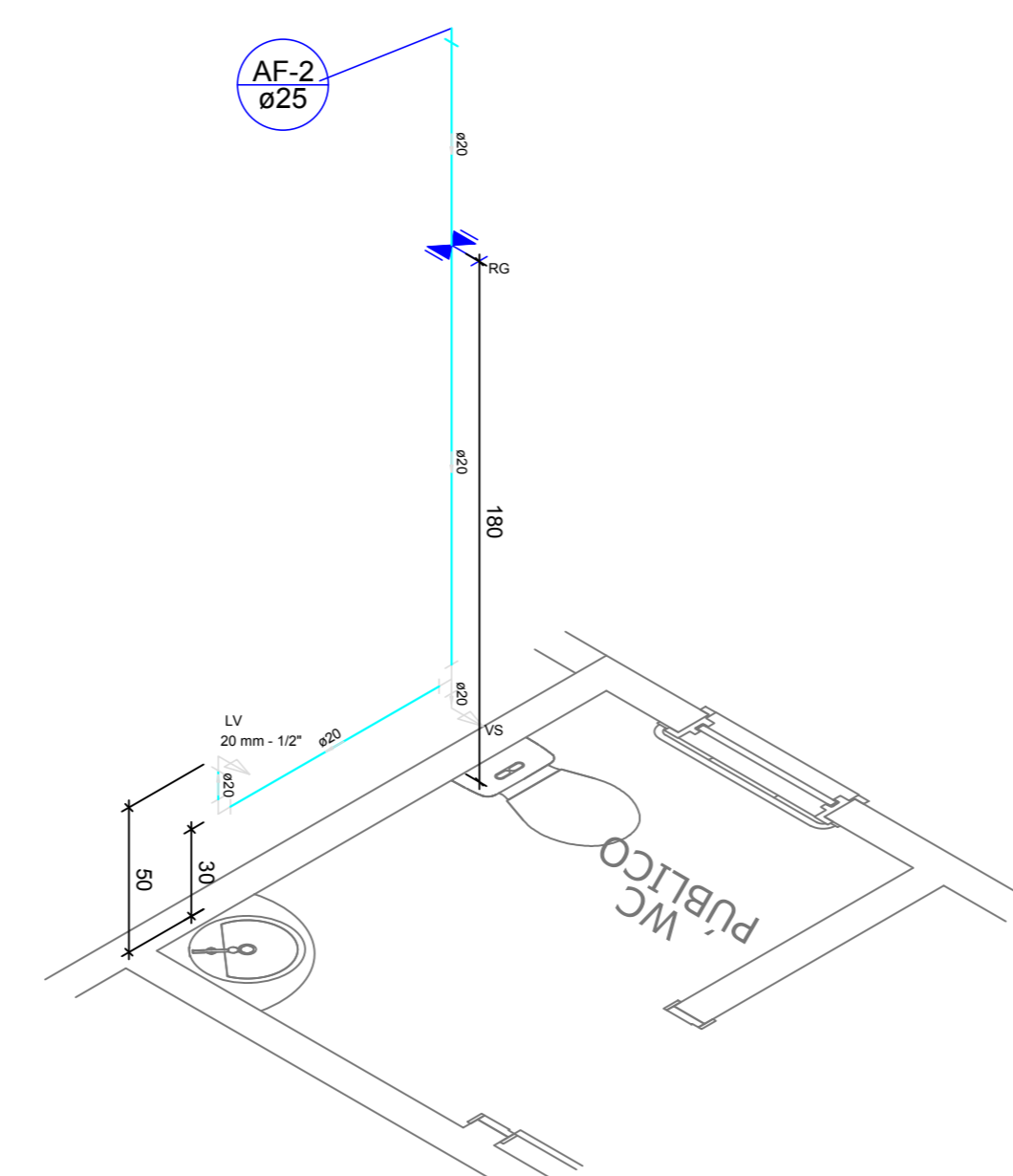
Detalhe ISOMÉTRICO BANHEIRO PÚBLICO escala 1:25
