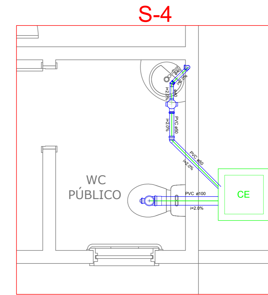
S-4 (Detalhe Sanitário BANHEIRO PÚBLICO) escala 1:25
