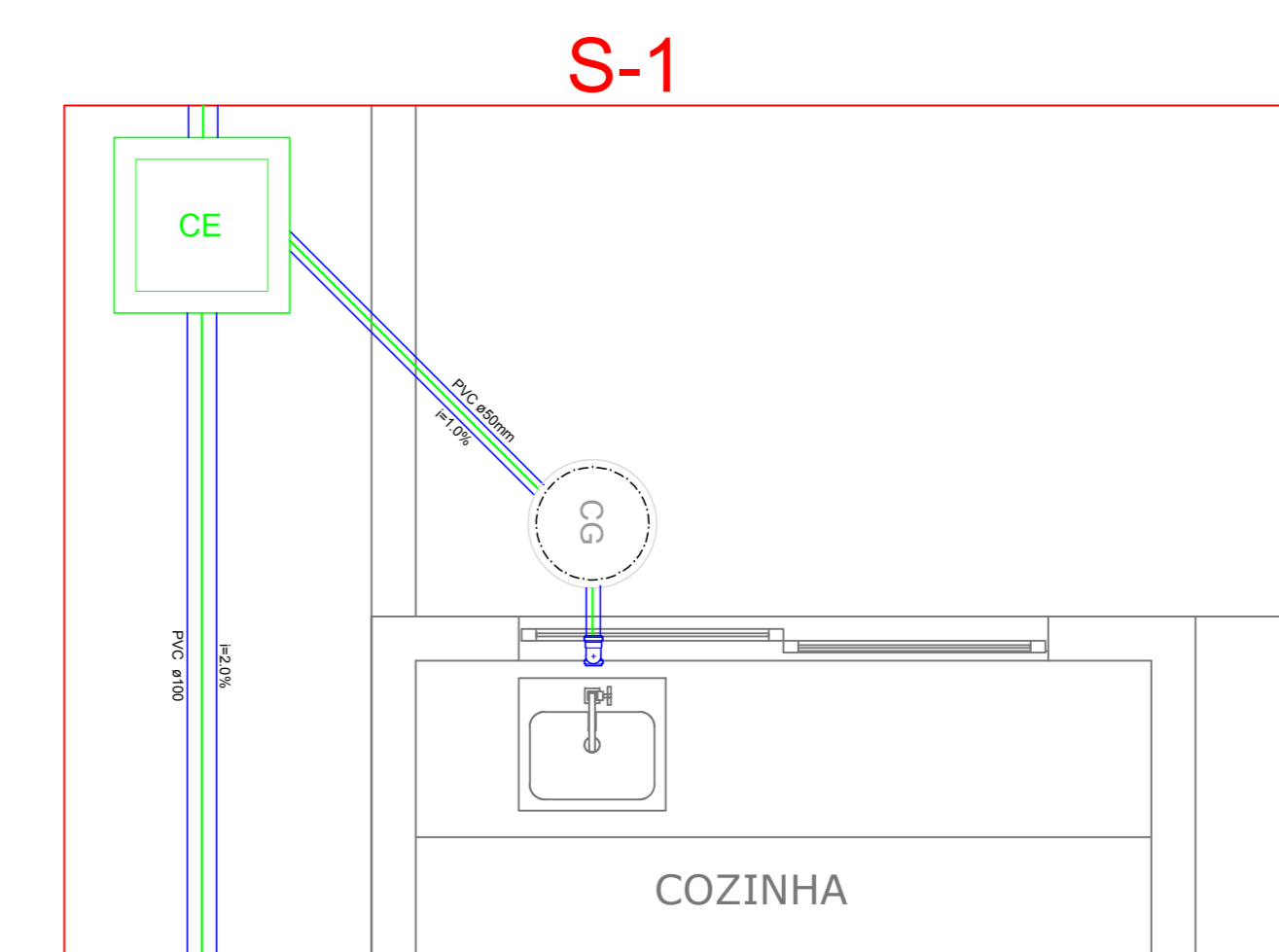
S-1 (Detalhe Sanitário COZINHA) escala 1:25
