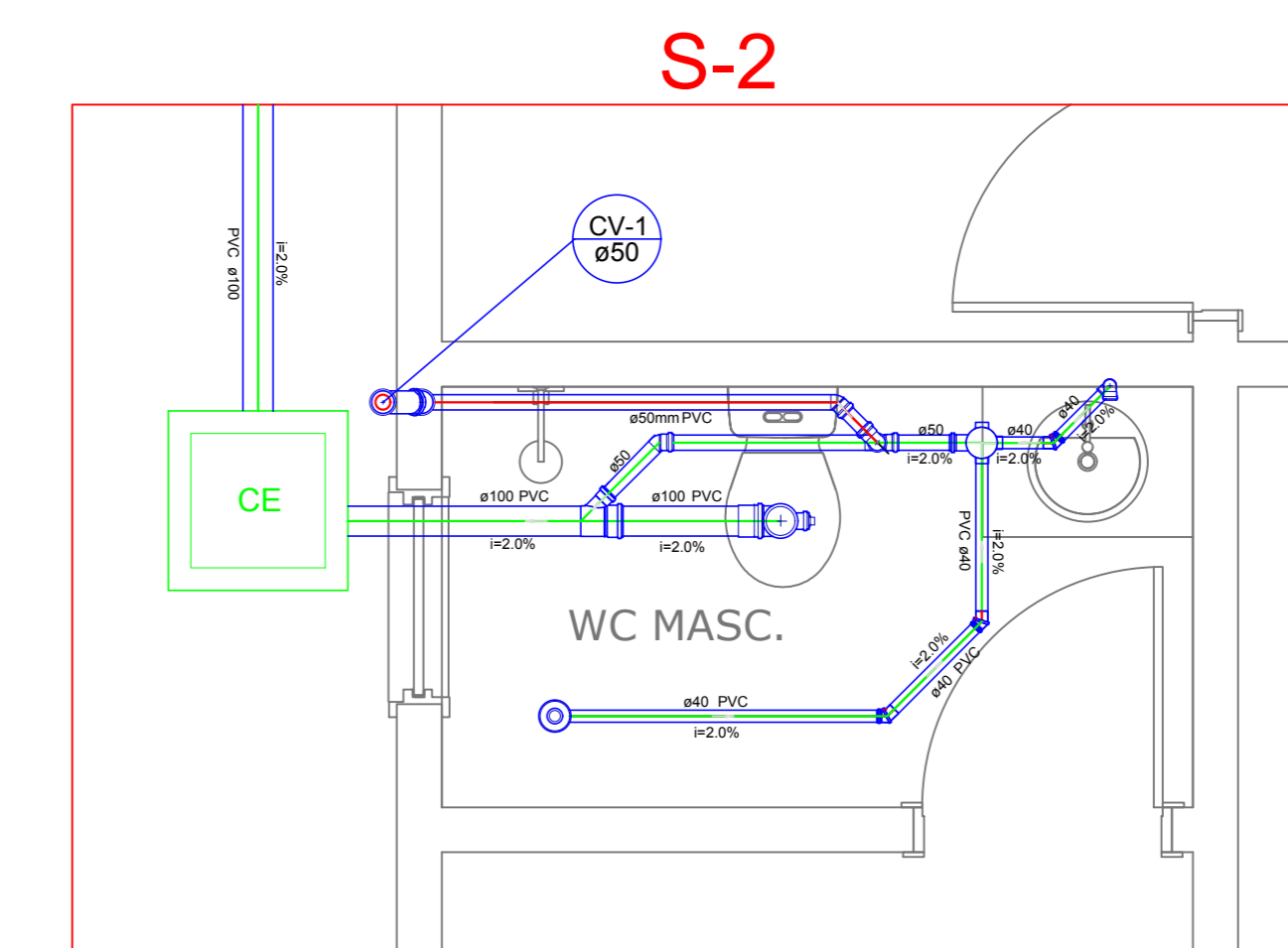
S-2 (Detalhe Sanitário BANHEIRO BANHO MASC.) escala 1:25
