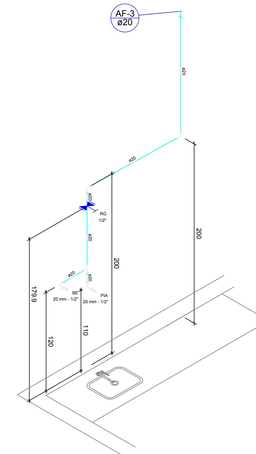
Detalhe COZINHA escala 1:25
