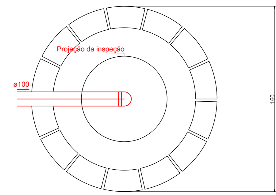
SUMIDOURO - PLANTA BAIXA S/ ESC.
