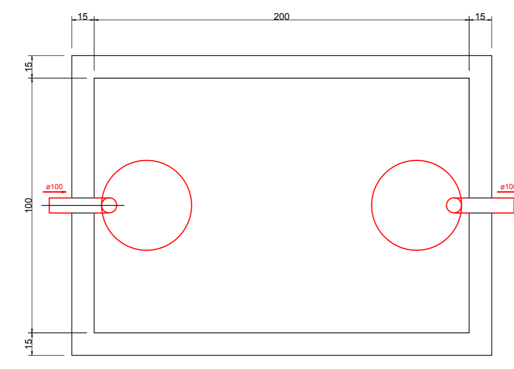
TANQUE SÉPTICO - PLANTA BAIXA S/ ESC.
