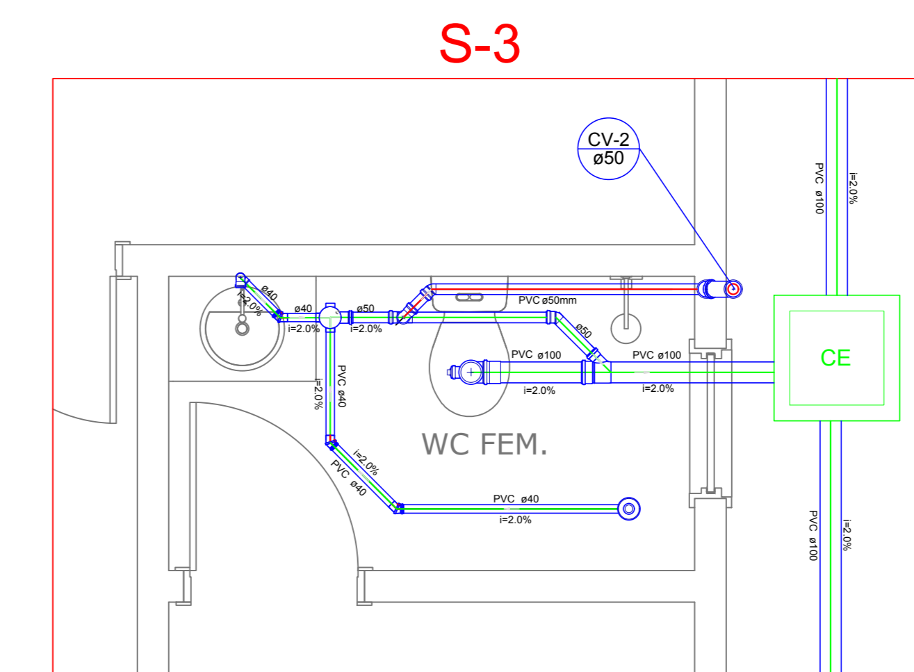
S-3 (Detalhe Sanitário BANHEIRO BANHO MASC.) escala 1:25
