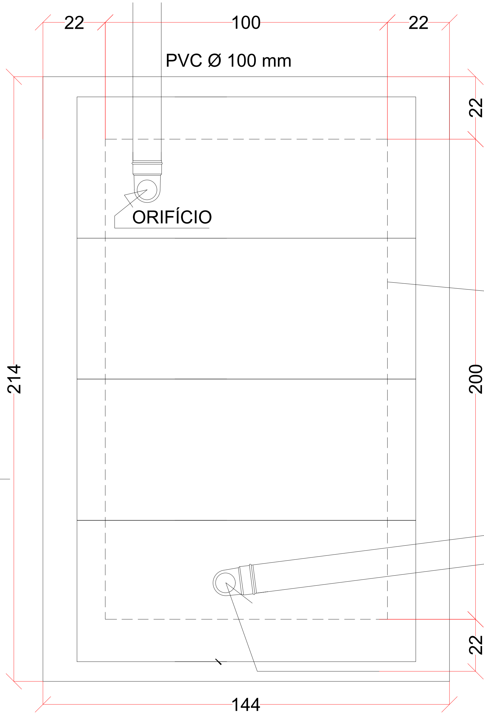
TANQUE SÉPTICO PLANTA BAIXA ESC. 1:30
