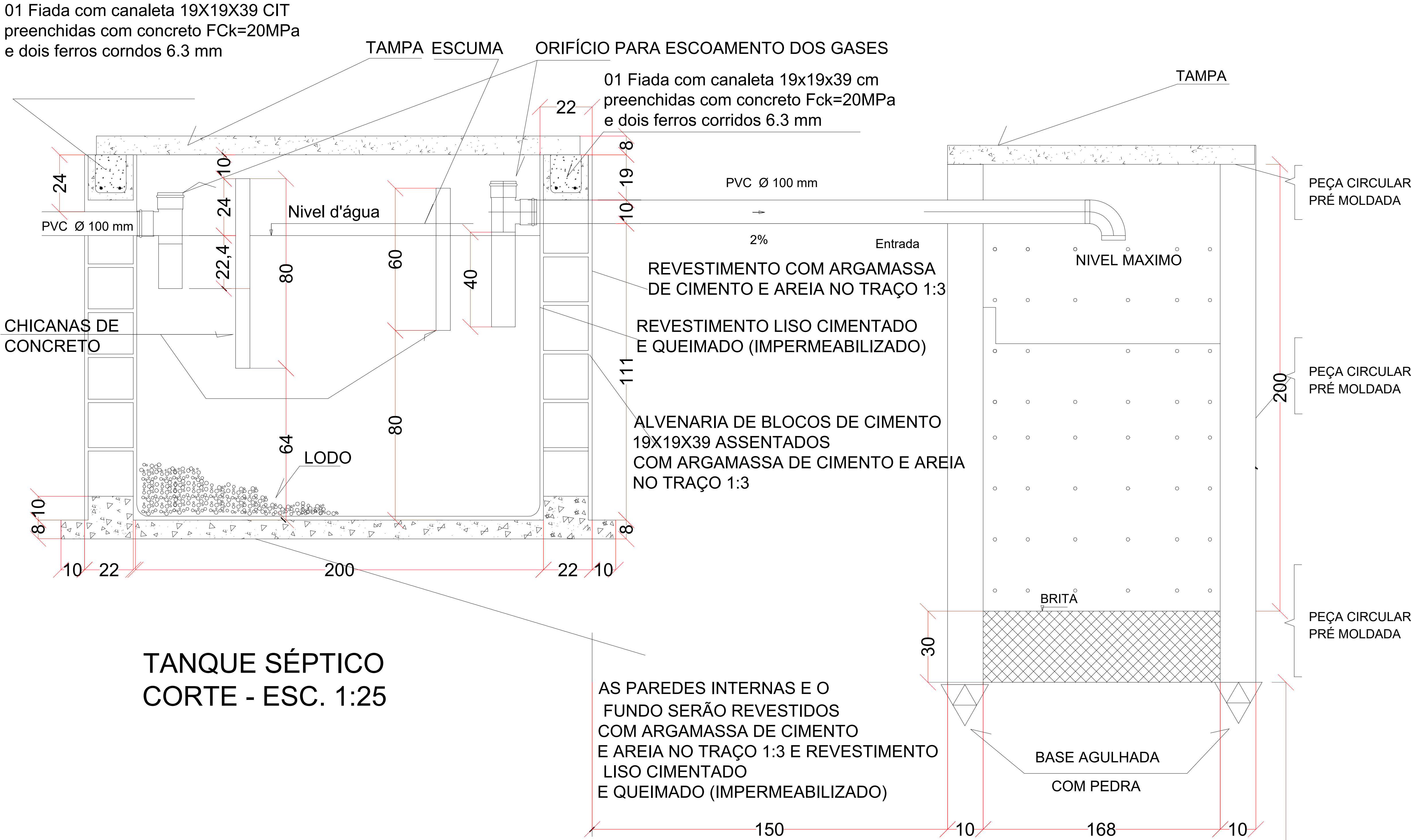
SUMIDOURO CORTE AA-ESC. 1:25
